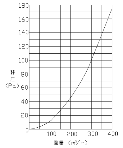
圧損特性
